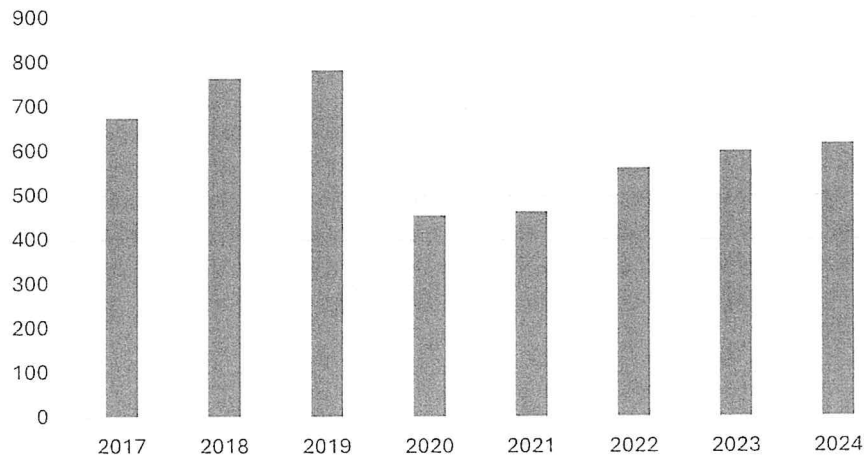
Evolution adhérents 2017-2024
